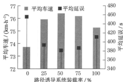
图 6 不同路径诱导系统装载率下的平均车速和延误对比
