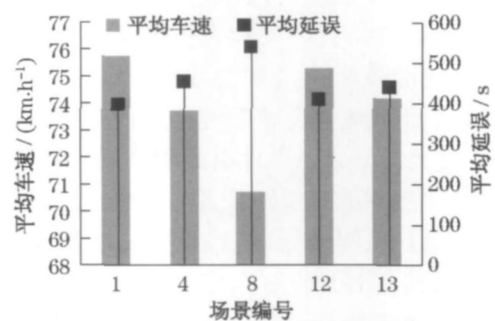
图5 路径诱导系统下的平均车速和平均延误对比
